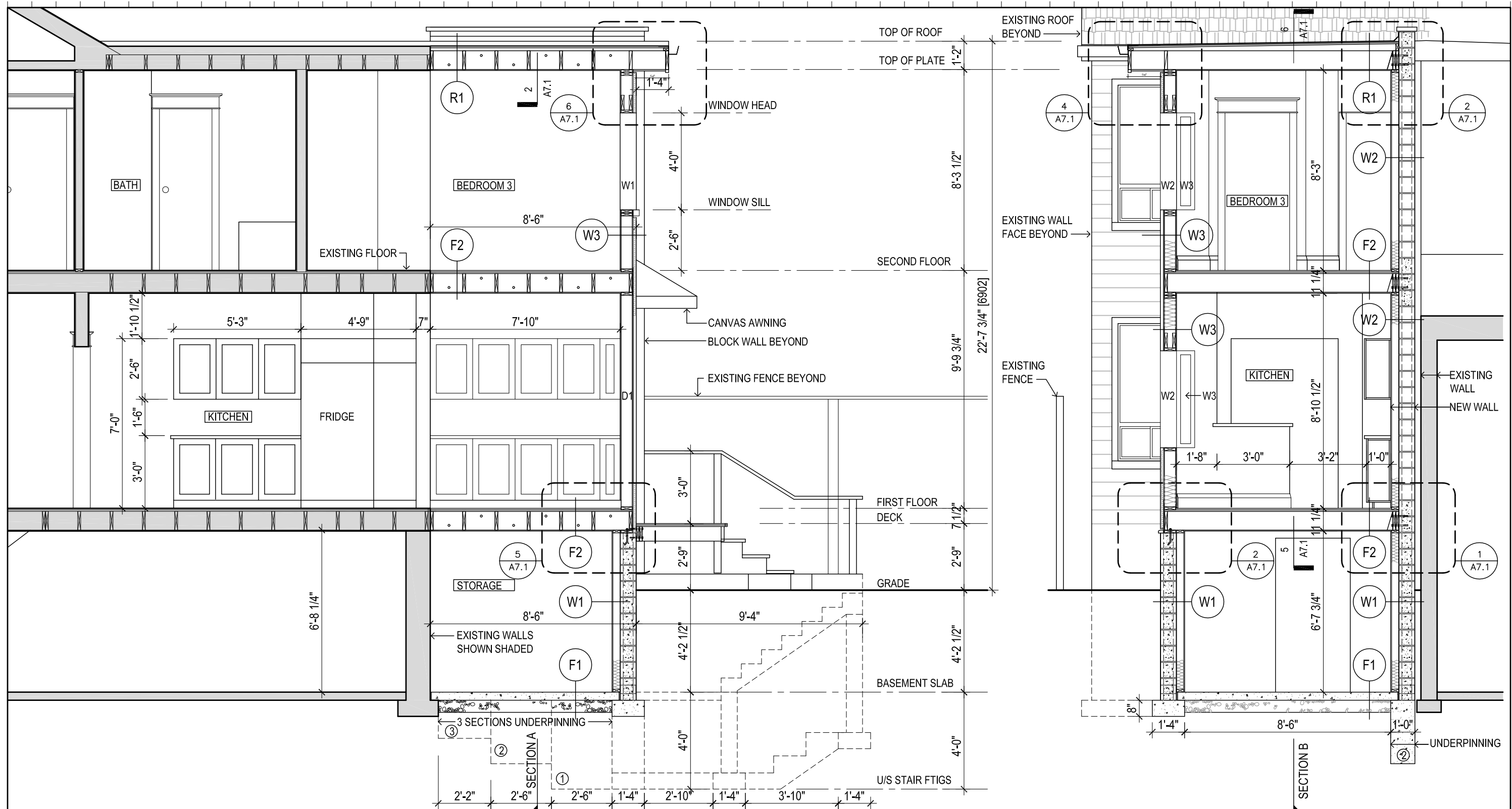
2 Section B A7 Scale: 1/4"=1'-0"
