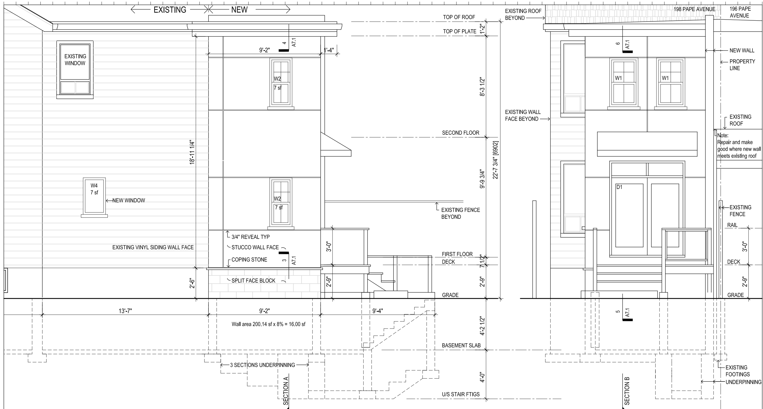
1 North Elevation A6 Scale: 1/4"=1'-0" 1 A7
