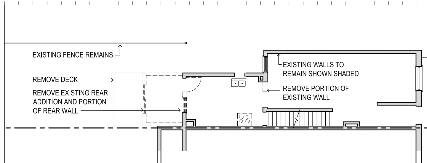
2 First Floor Existing A3 Scale: 1" = 10'-0"
